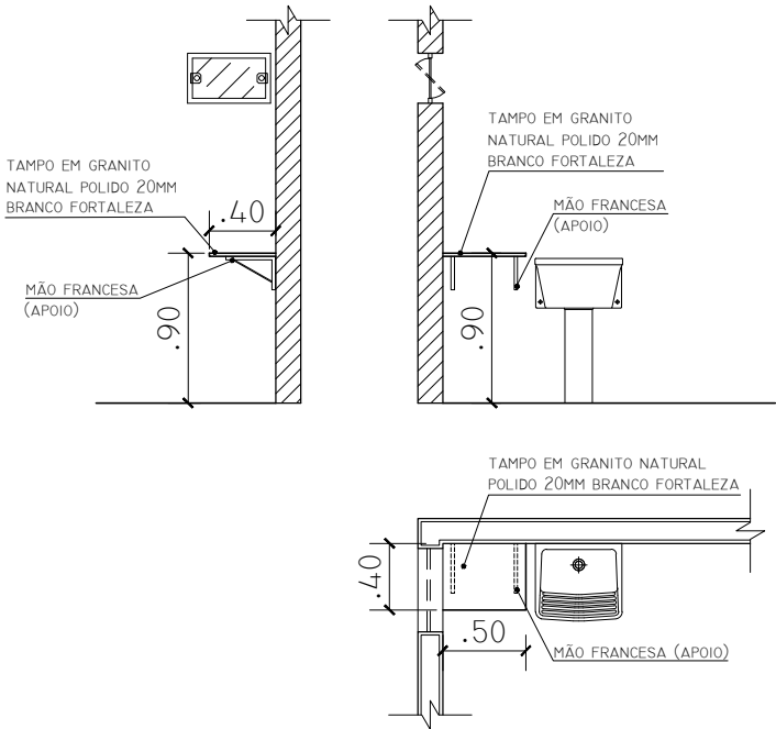
ÁREA DE SERVIÇO ESC. 1:50
