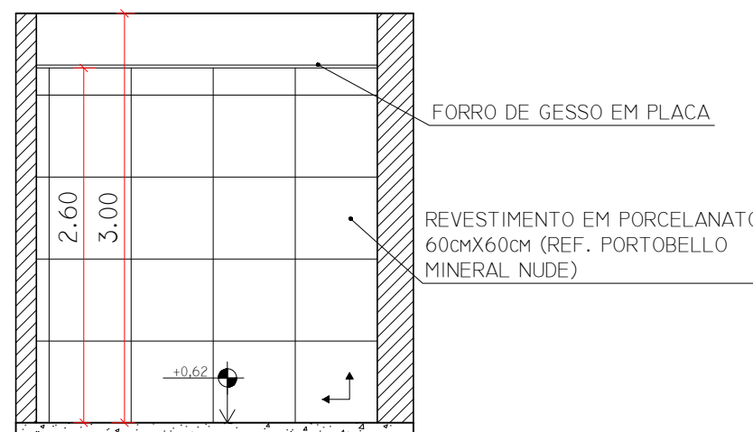
WC PNE - VISTA D
