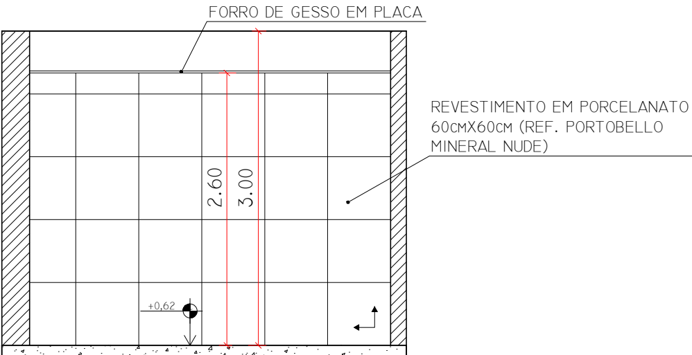
COPA - VISTA C
