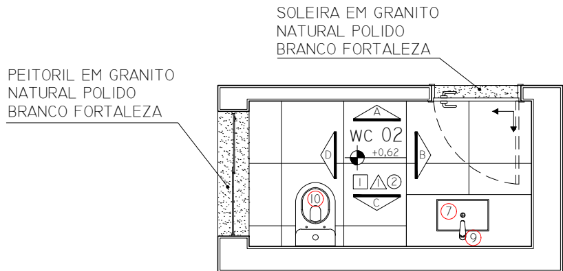
WC 02 - PLANTA BAIXA
