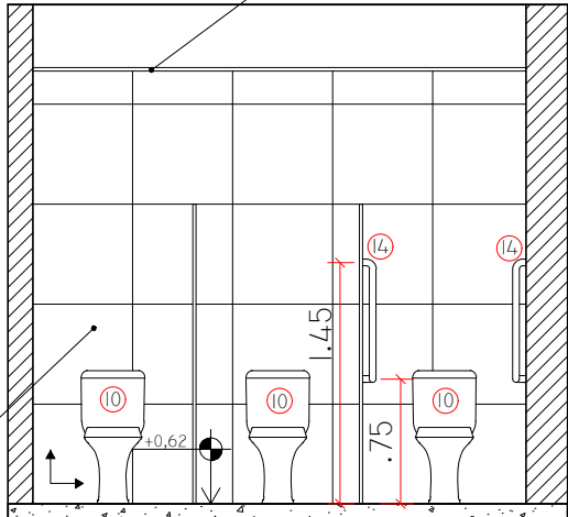
WC FEM. - VISTA D
