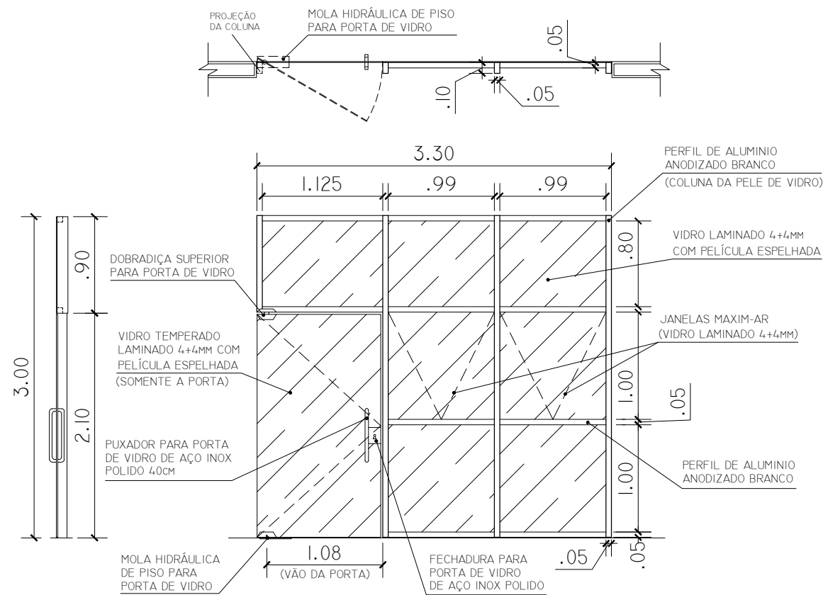
PELE DE VIDRO COM PORTA ESC. 1:50
