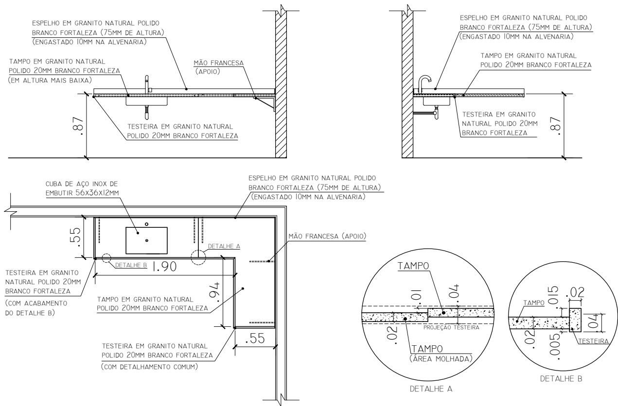
COPA ESC. 1:50
