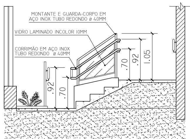
CORTE C-C ESC. 1:50
