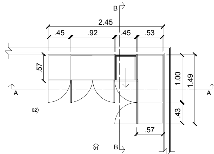
PLANTA BAIXA ARMÁRIO INFERIOR ESC. 1:50
