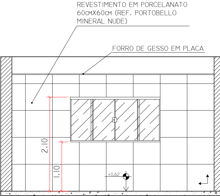
COPA - VISTA B
