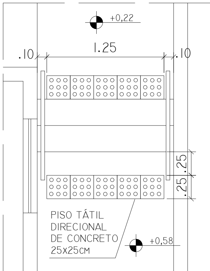
DETALHE 05 ESC. 1:25
