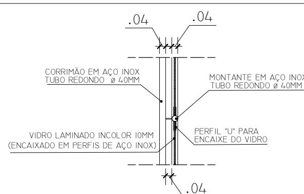
DETALHE - SEÇÃO HORIZONTAL ESC. 1:50
