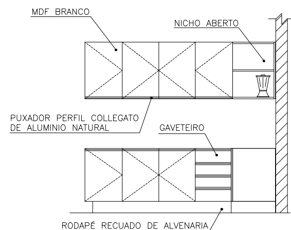
VISTA 1 ESC. 1:50
