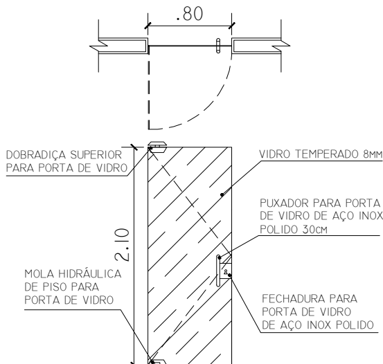
PORTA P5 ESC. 1:50
