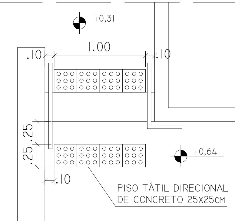
DETALHE 04 ESC. 1:25
