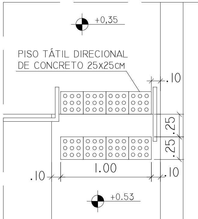
DETALHE 03 ESC. 1:25
