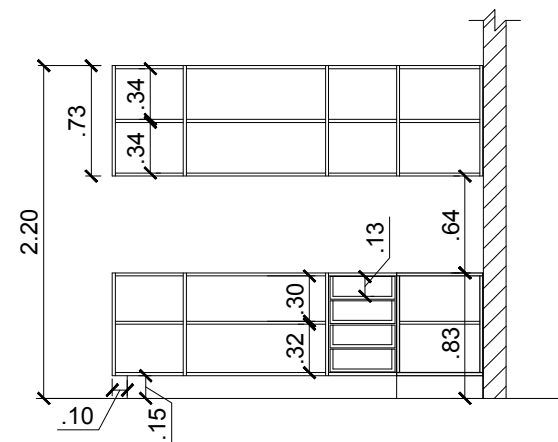
CORTA AA ESC. 1:50
