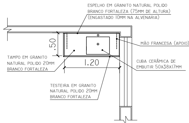
WC PROCURADOR 01 ESC. 1:50
