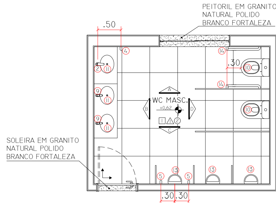
WC MASC. - PLANTA BAIXA
