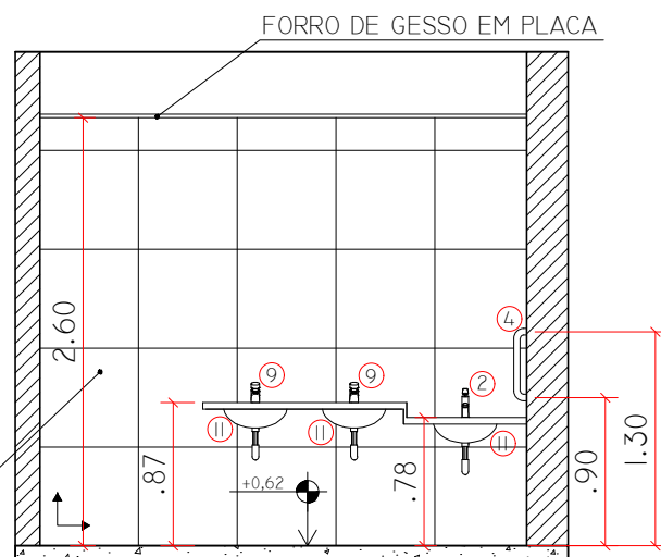
WC MASC. - VISTA D
