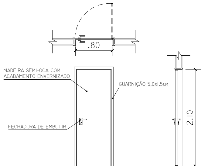
PORTA P1 ESC. 1:50
