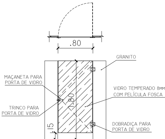
PORTA P6 ESC. 1:50
