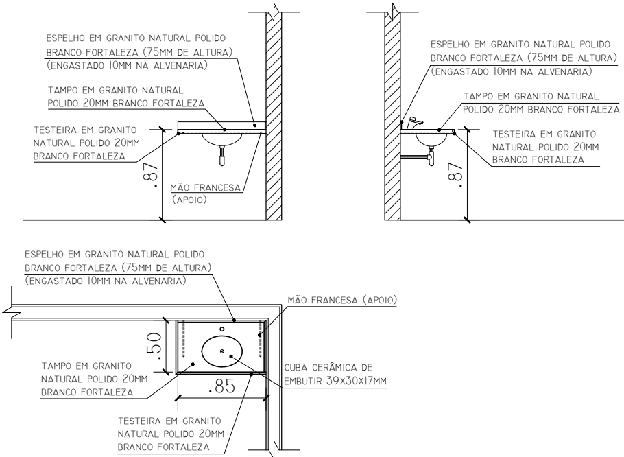
WBC (ÁREA DE SERVIÇO) ESC. 1:50
