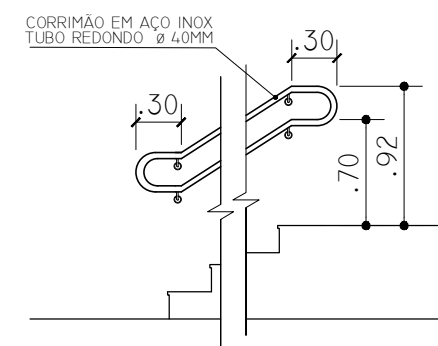
VISTA - CORRIMÃO FIXADO NA PAREDE ESC. 1:50
