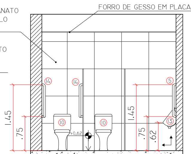
WC MASC. - VISTA B
