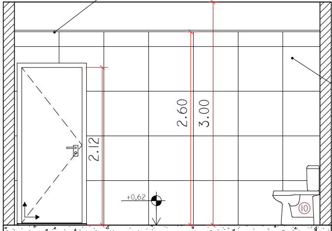
WC FEM. - VISTA C
