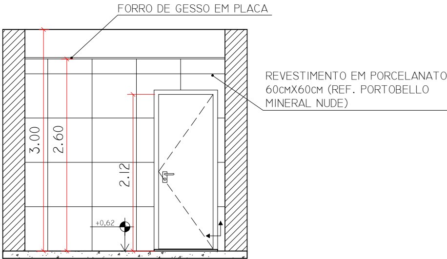
WC 02 - VISTA A
