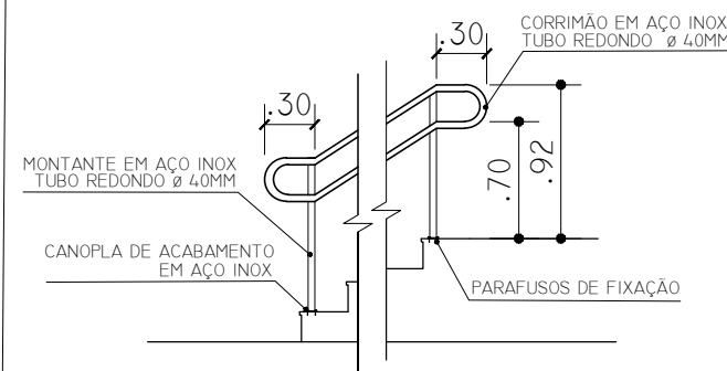
VISTA - CORRIMÃO APOIADO EM MONTANTE ESC. 1:50
