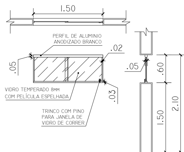
JANELA J2 ESC. 1:50
