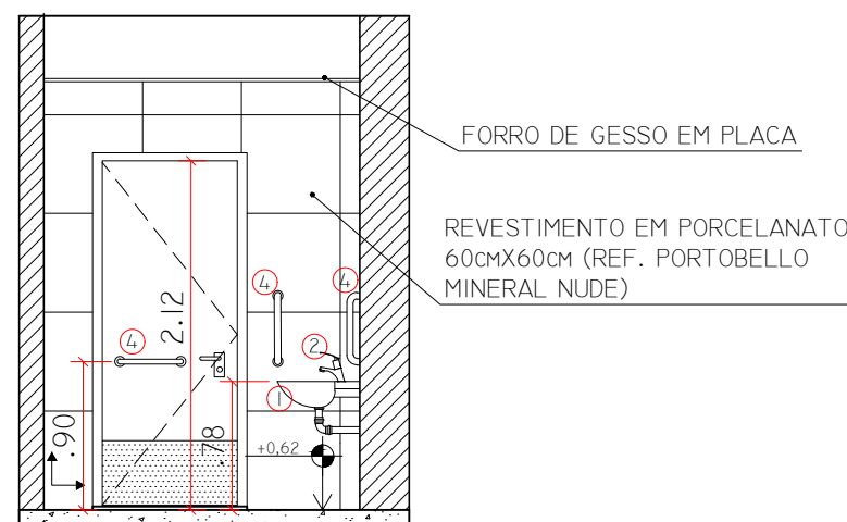
WC PNE - VISTA A
