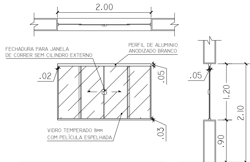
JANELA J1 ESC. 1:50
