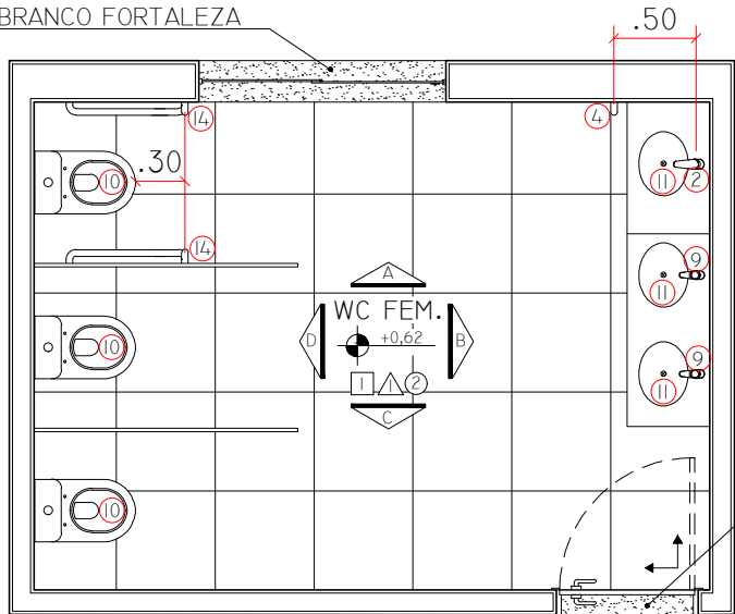
WC FEM. - PLANTA BAIXA
