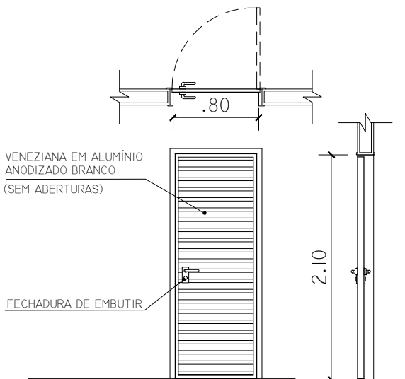
PORTA P3 ESC. 1:50
