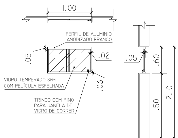
JANELA J3 ESC. 1:50
