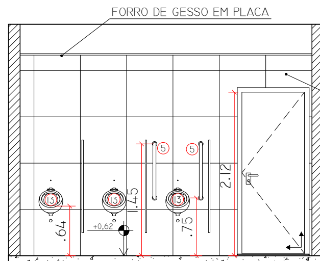
WC MASC. - VISTA C
