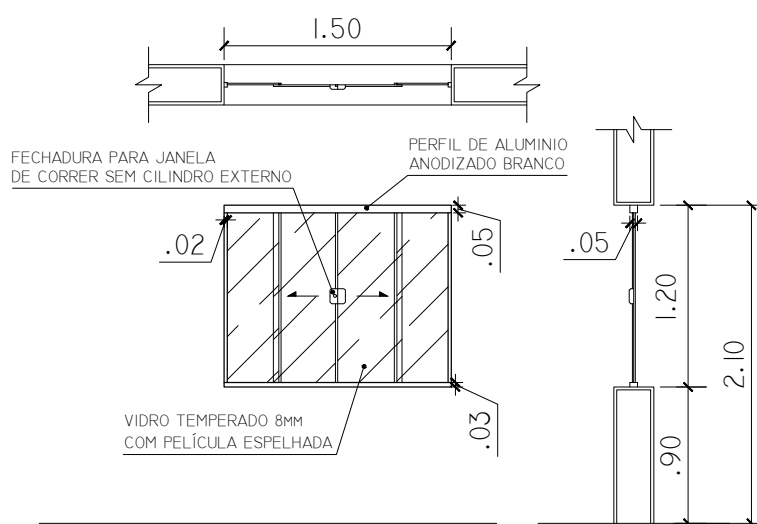
JANELA J5 ESC. 1:50
