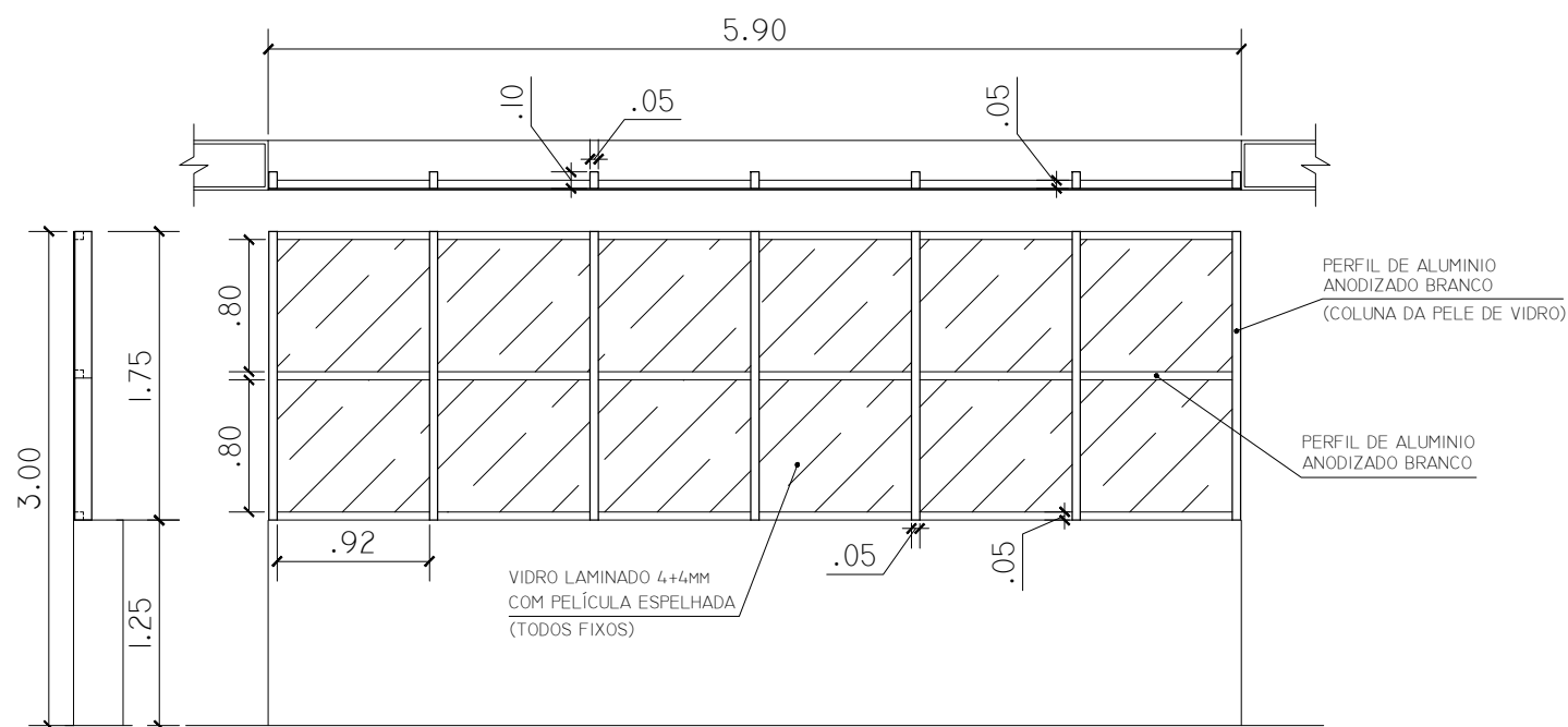
PELE DE VIDRO ESC. 1:50
