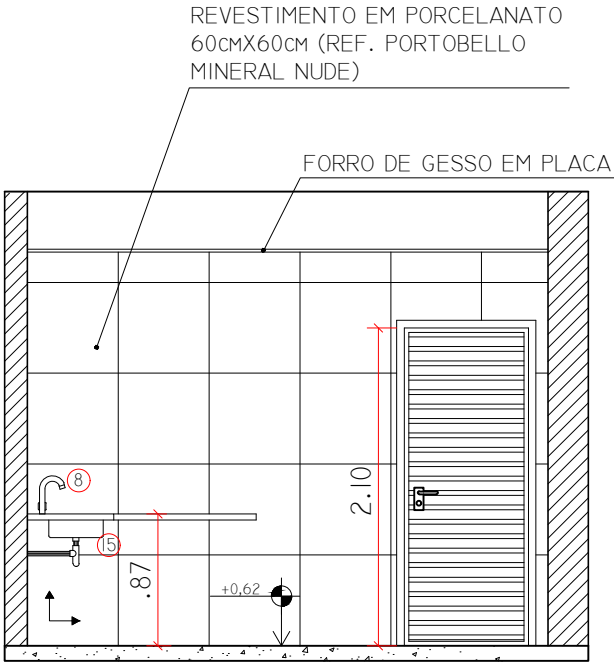
COPA - VISTA A
