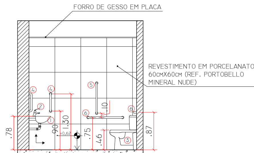
WC PNE - VISTA B
