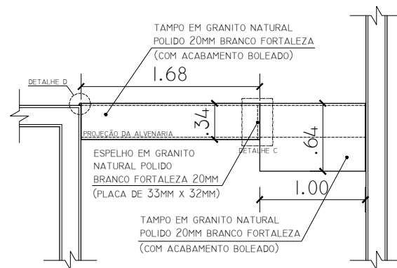
BALCÃO DE PROTOCOLO ESC. 1:50
