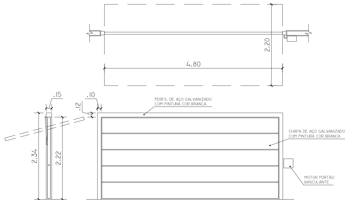
PORTÃO BASCULANTE ESC. 1:50
