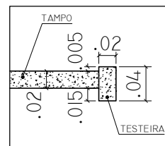
DETALHE DO ACABAMENTO
