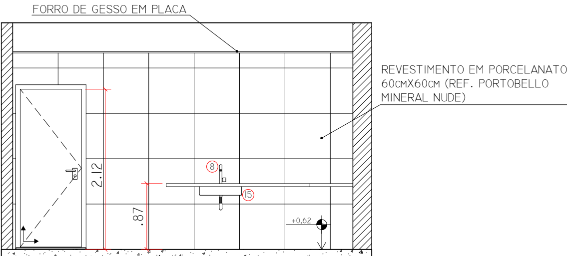
COPA - VISTA D
