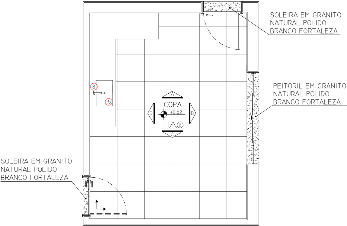
COPA - PLANTA BAIXA
