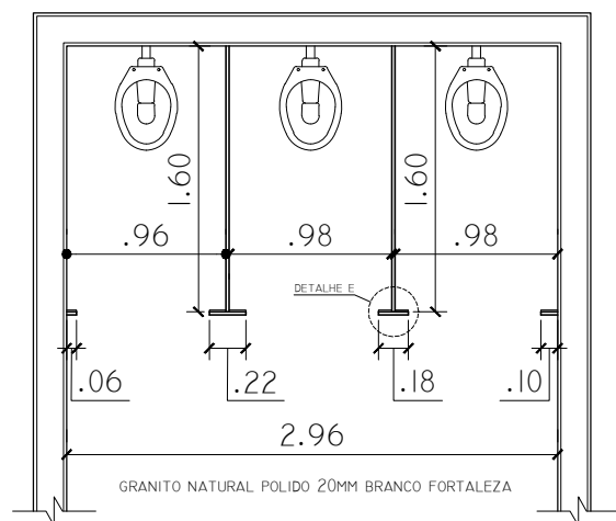
BOXES WC FEM. ESC. 1:50
