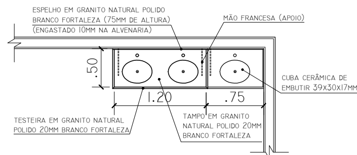
WC MASC. / WC FEM. ESC. 1:50
