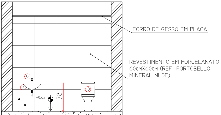
WC 02 - VISTA C
