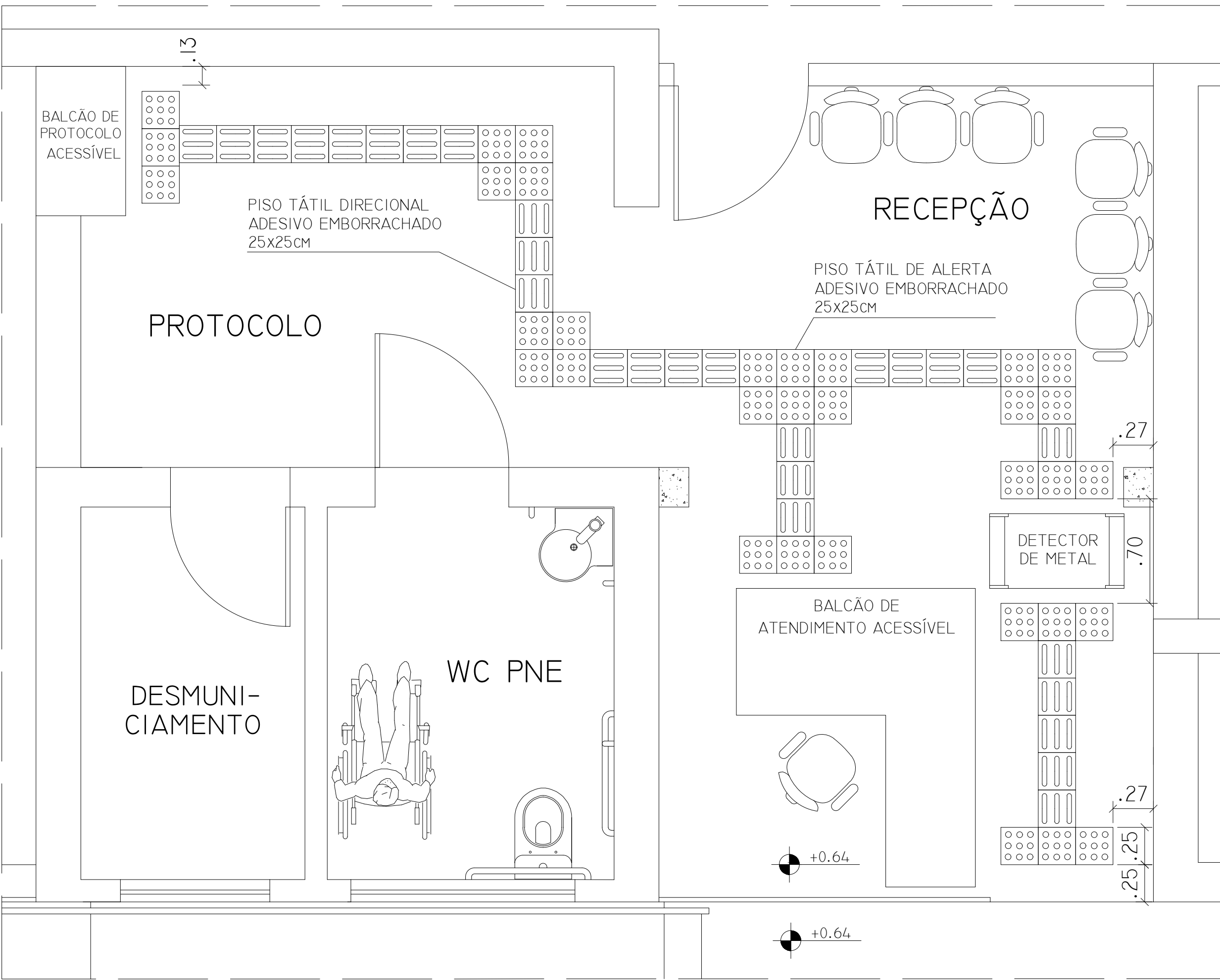
DETALHE 02 ESC. 1:25
