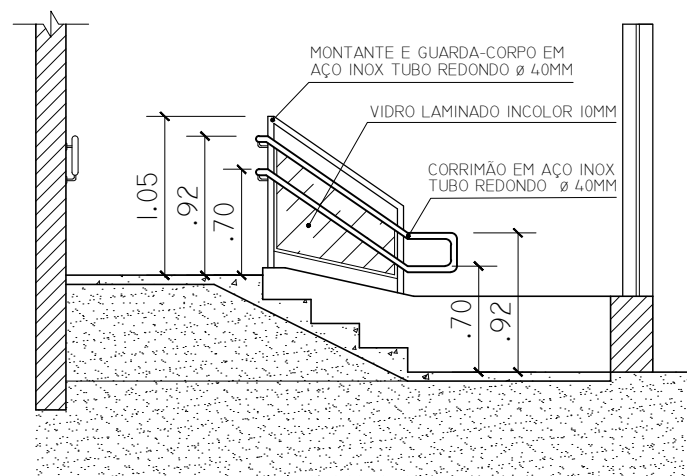
CORTE D-D ESC. 1:50
