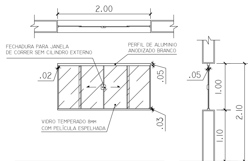
JANELA J4 ESC. 1:50
