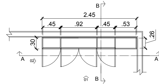
PLANTA BAIXA ARMÁRIO SUPERIOR ESC. 1:50
