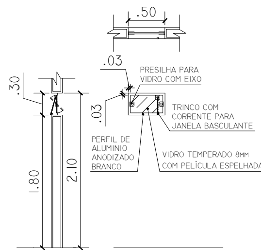
JANELA J6 ESC. 1:50
