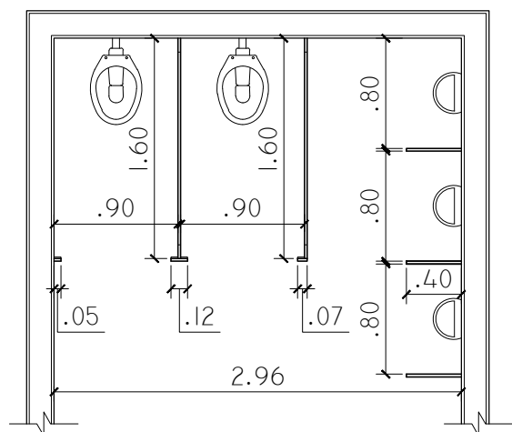
BOXES WC MASC. ESC. 1:50
