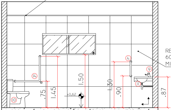
WC FEM. - VISTA A
