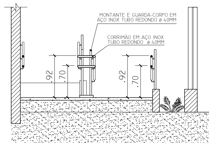
CORTE E-E ESC. 1:50
