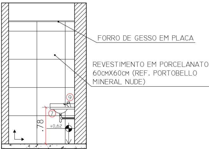
WC 02 - VISTA B
