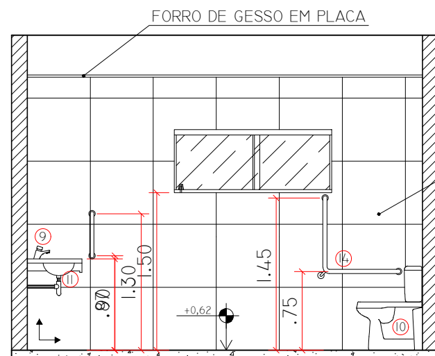
WC MASC. - VISTA A
