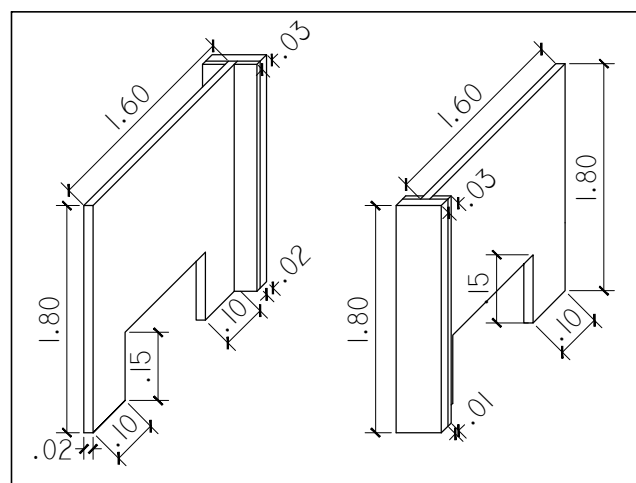
ESQUEMA 3D - DIVISÓRIAS DO WC
