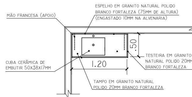
WC PROCURADOR 02 ESC. 1:50
