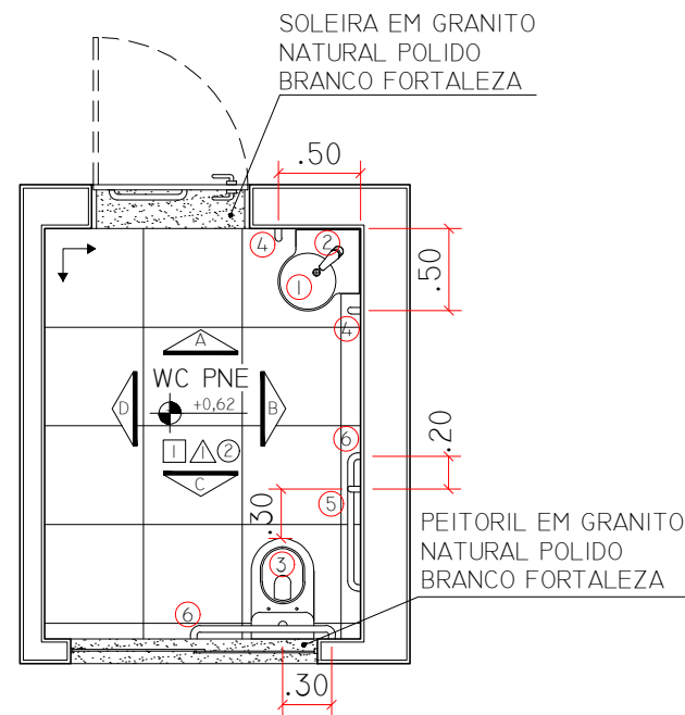
WC PNE - PLANTA BAIXA
