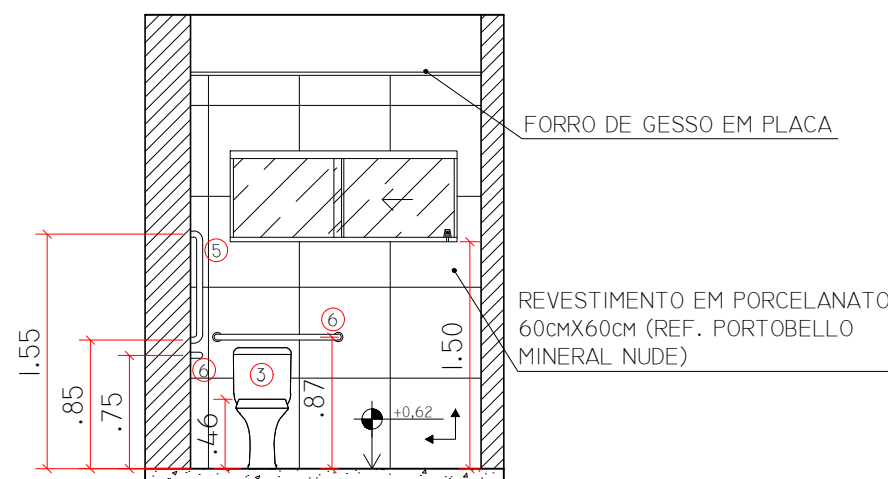
WC PNE - VISTA C
