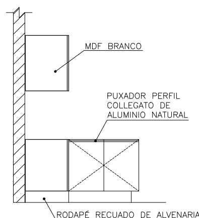
VISTA 2 ESC. 1:50
