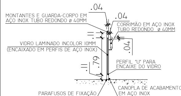
DETALHE - SEÇÃO VERTICAL ESC. 1:50
