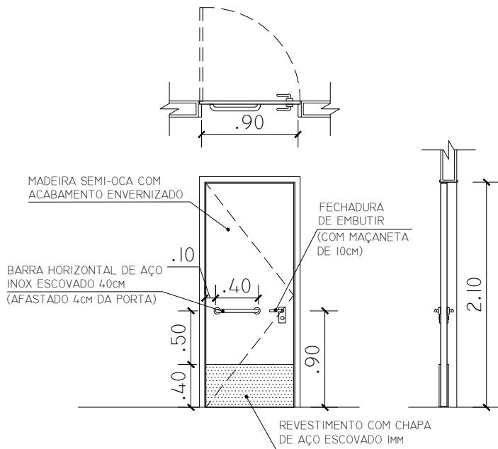
PORTA P2 ESC. 1:50
