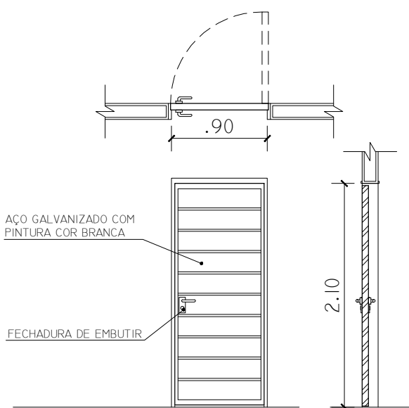
PORTA P4 ESC. 1:50
