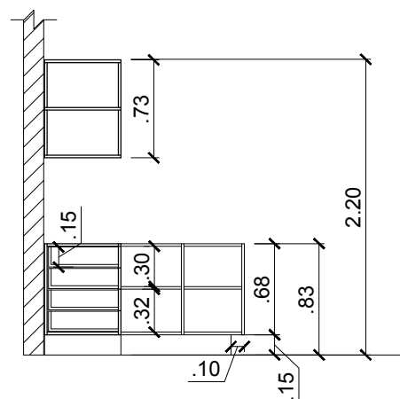
CORTA BB ESC. 1:50
