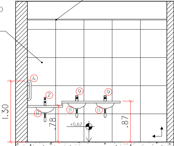
WC FEM. - VISTA B
