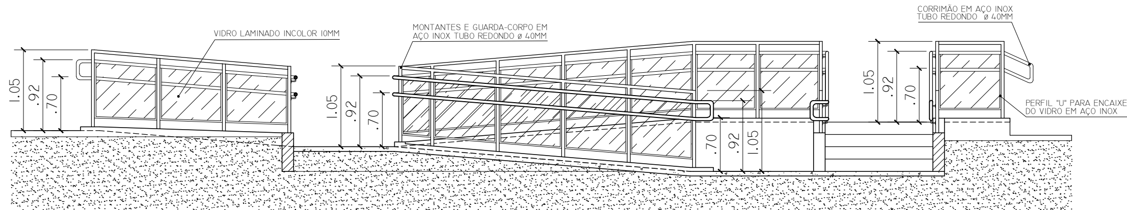
CORTE B-B ESC. 1:50
