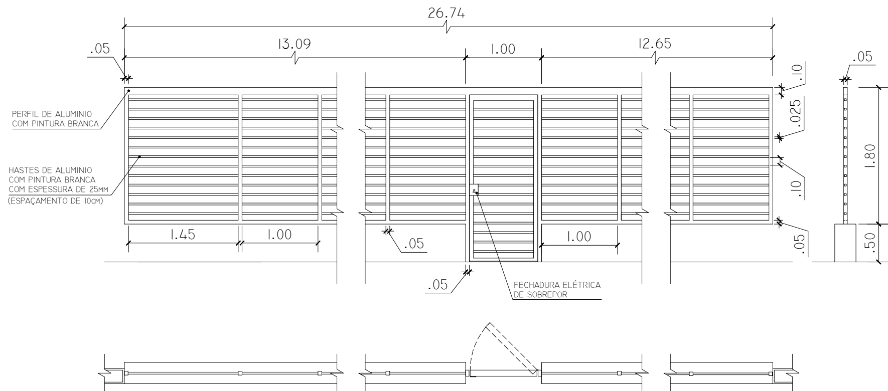
GRADIL FRONTAL ESC. 1:50
