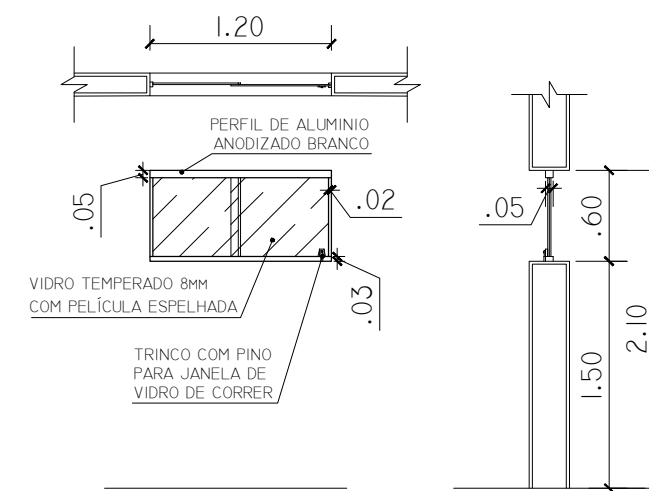
JANELA J7 ESC. 1:50
