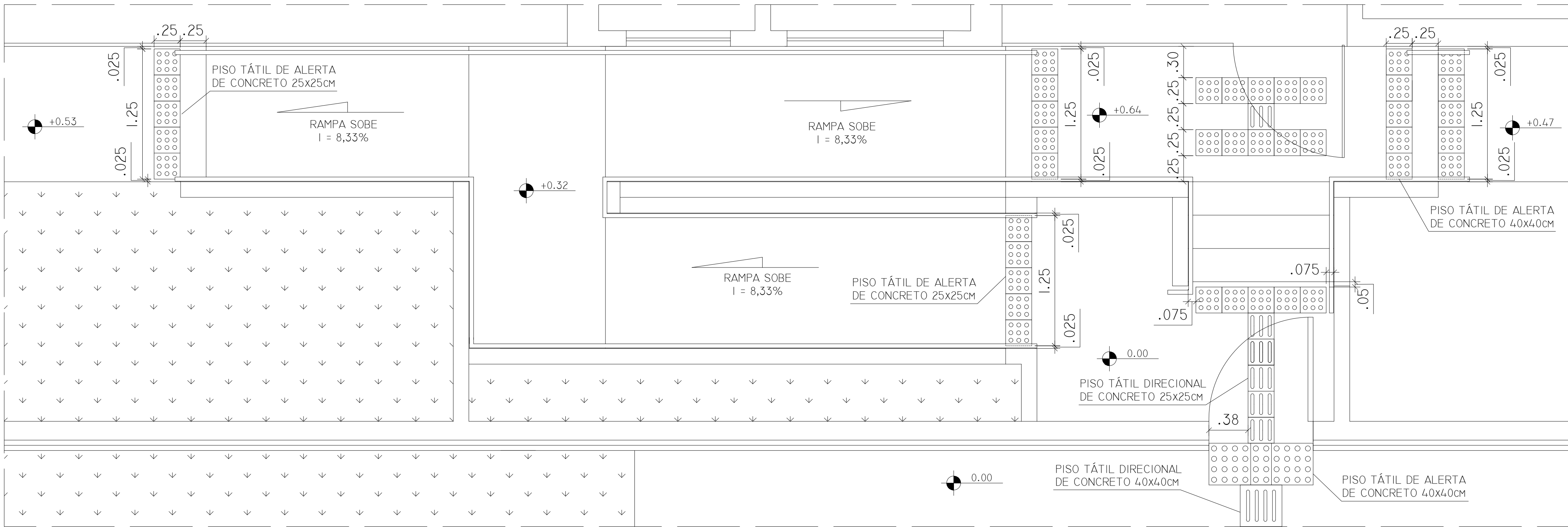
DETALHE 01 ESC. 1:25
